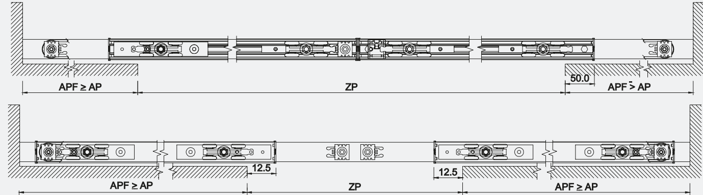
PLANTA SISTEMA ABIERTO / CERRADO
