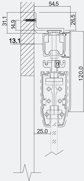
Fijación lateral conector muro ancho
