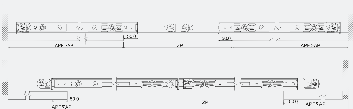
ELEVACIÓN SISTEMA CERRADO PAÑO FIJO VIDRIO
