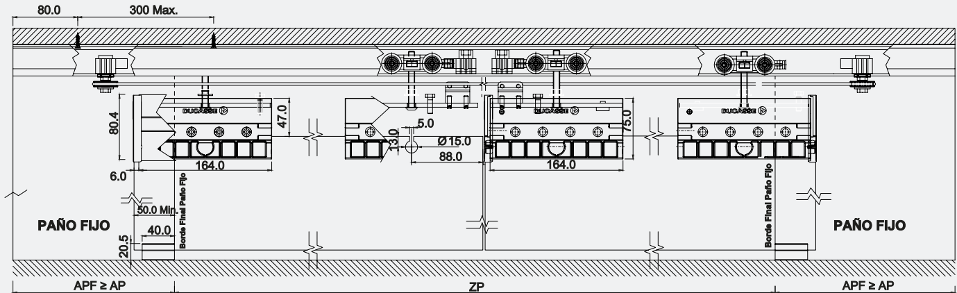
ELEVACIÓN SISTEMA CERRADO PAÑO FIJO MURO
