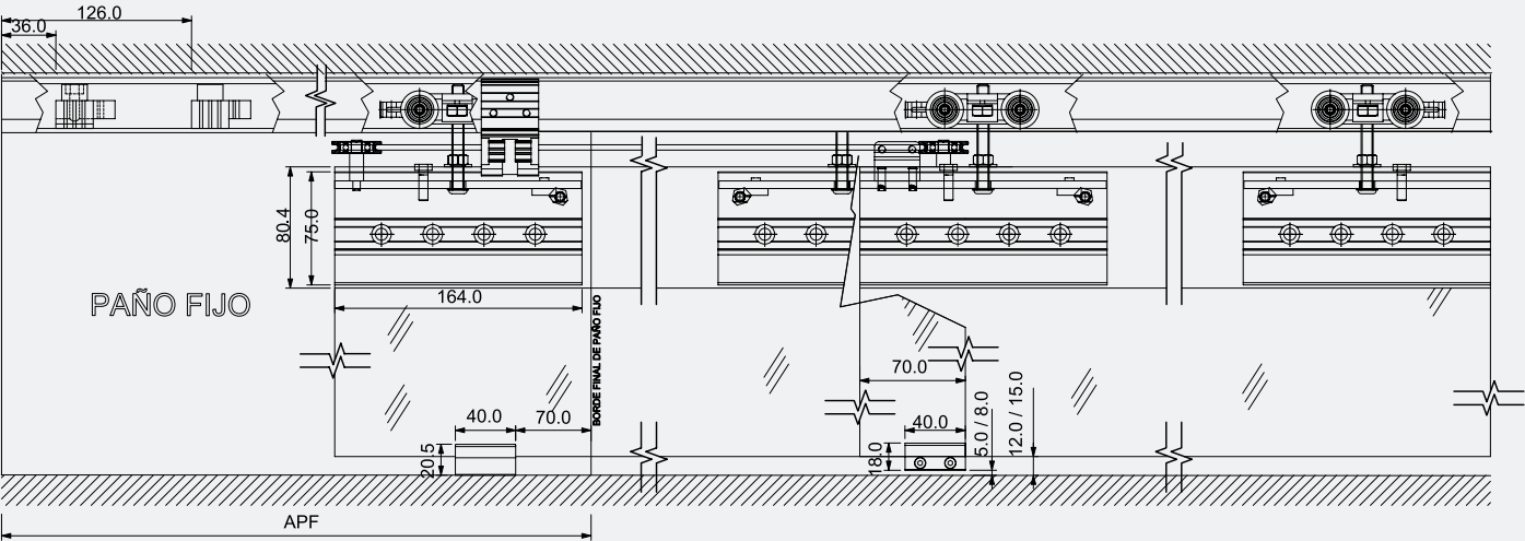
ELEVACIÓN SISTEMA CERRADO PAÑO FIJO MURO
