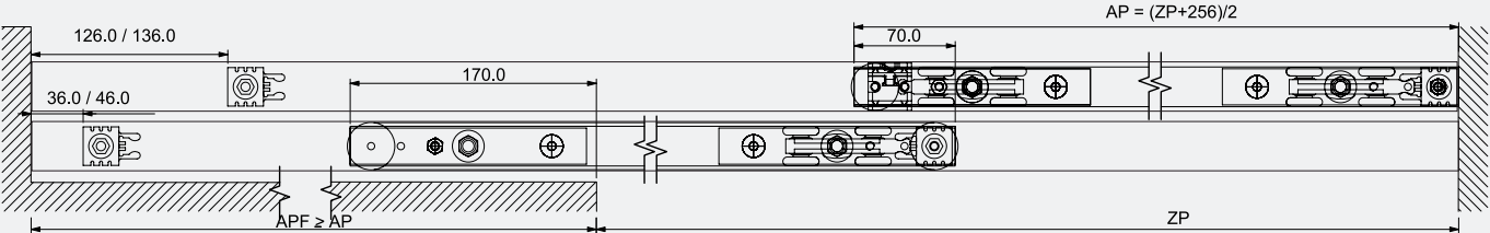
PLANTA SISTEMA ABIERTO / CERRADO
