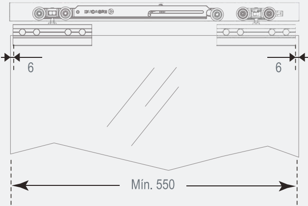
Easy Soft DN80 + Kit anexo ES DN80 VD + Mordaza Perforada e = 8-10mm | 12-13mm
