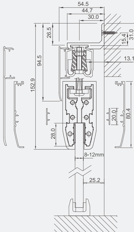
Fijación muro ancho
