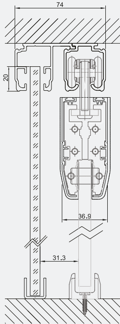
Fijación riel paño fijo
