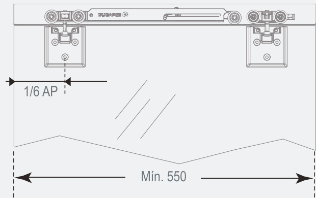
Easy Soft DN80 + Kit anexo ES DN80 VD + Mordaza Perforada e = 8-10mm | 12-13mm
