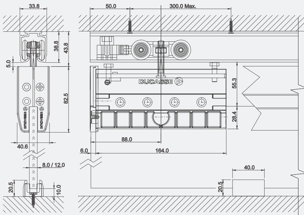
Fijación cielo
