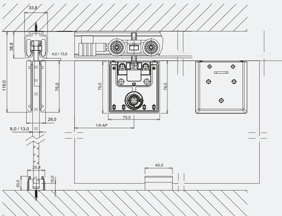
Fijación cielo
