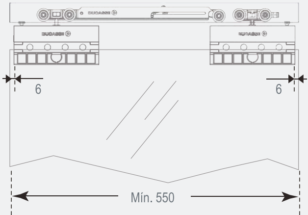
Easy Soft DN80 + Kit anexo ES DN80 VD + Mordaza Pres/Perf e = 8-10mm | 12-13mm
