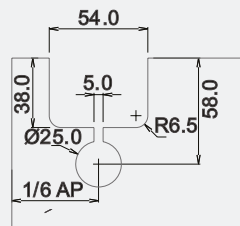
Detalle mecanizado vidrio
