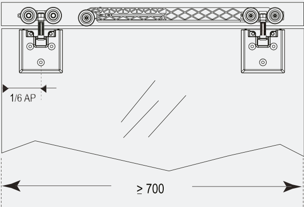
ES DN150 + Kit anexo ES DN150 + Mordaza Perforada e = 8-10mm | 12-13mm
