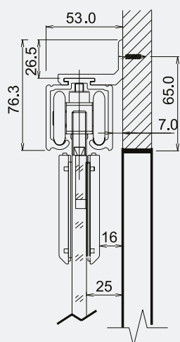
Fijación muro
