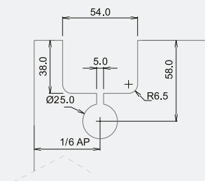
Detalle Mecanizado Vidrio
