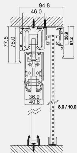
Opción con riel paño fijo
