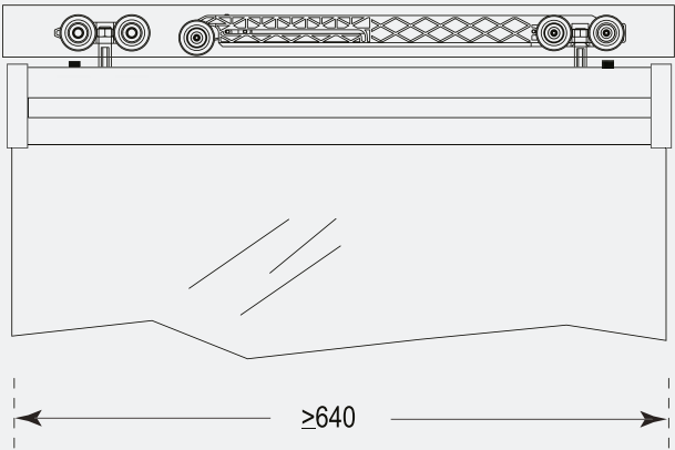
Instalación con Mordaza Pres/Perf:
