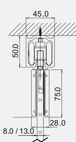
Fijación cielo
