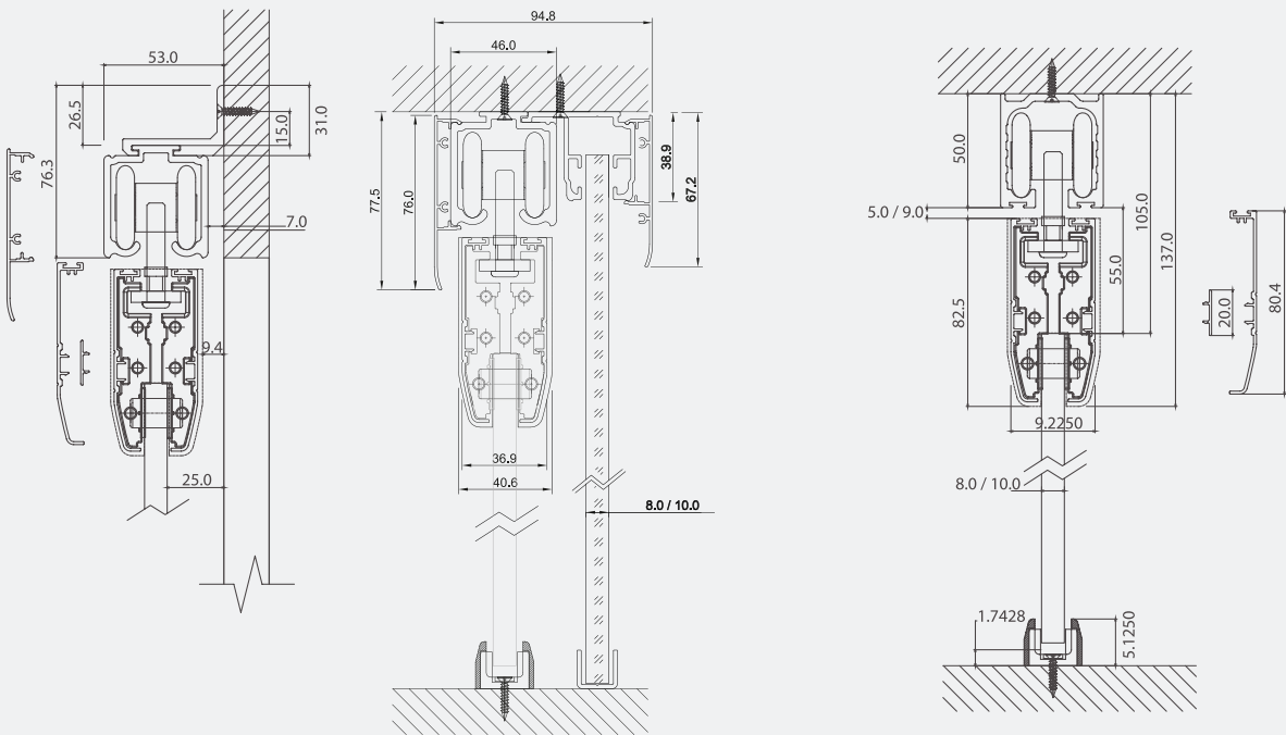
Fijación muro
