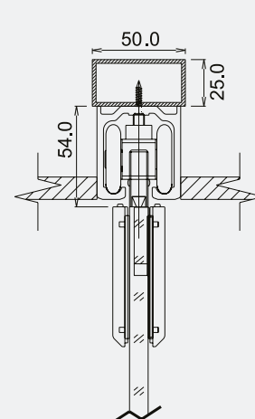
Fijación riel embutido
