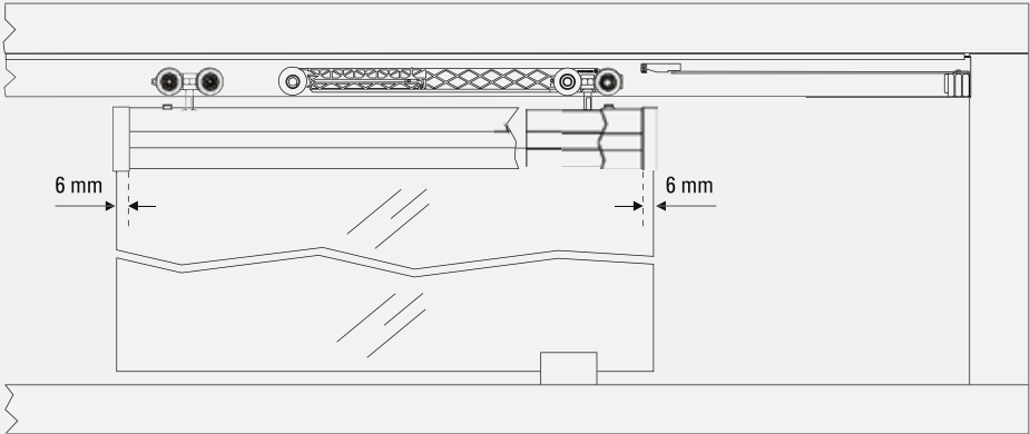
Instalación con Mordaza Pres/Perf:
